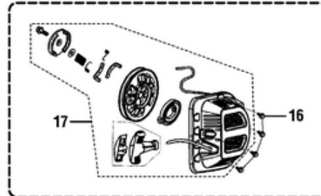
Recoil Starter Lanceur à rappel Arrancador retráctil
