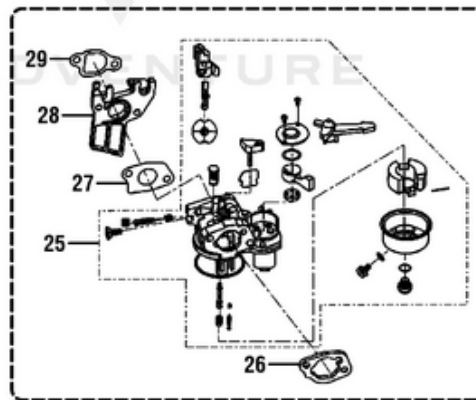
Carburetor Assembly Ensemble de carburateur Conjunto del carburador
