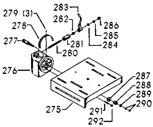
20-660 TILT TABLE
